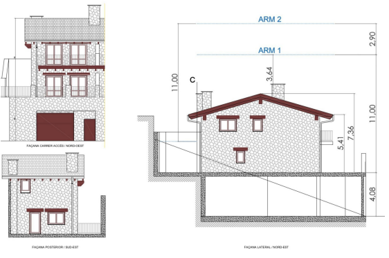
FAÇANA LATERAL / NORD-EST
